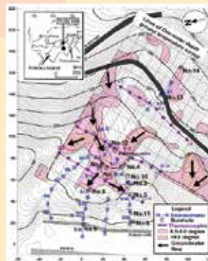
1 m深地温計測による自然斜面における地下水の流動経路の推定 (矢印が地下水の流れを示している)
