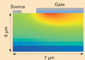
半導体素子内部の 温度分布シミュレーション
