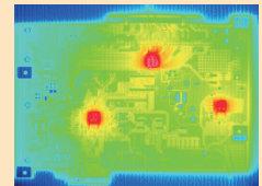
サーモグラフィを用いた プリント配線基板の温度分布計測
