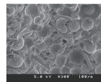
複合材料を作製して高熱伝導化を検証
