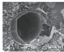
マイクロカプセルから接着剤を放出
