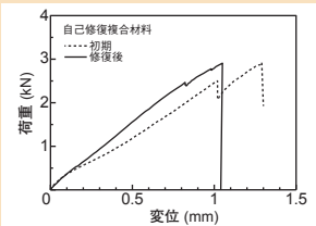
破壊した部分の再接着により強度が回復
