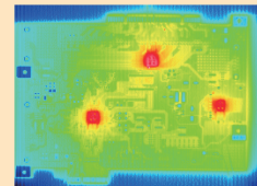
サーモグラフィを用いた プリント配線基板の温度分布計測
