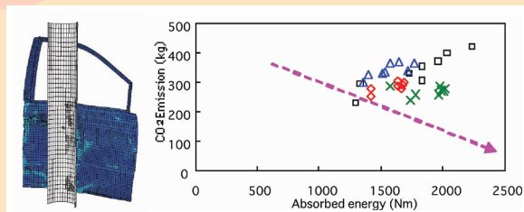
図1 ドアの側突解析 図2 ドアのCO 2 排出量とエネルギー吸収性能
