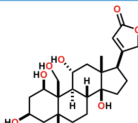
ウアバゲニン (Na + /K + -ATPase阻害剤のアグリコン)
