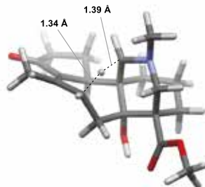
1,5-水素移動
