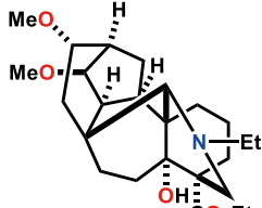
プベルリンCのモデル化合物
