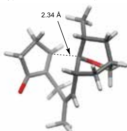
7-endo-ラジカル環化
