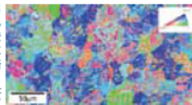
Fig. マグネシウム合金の室温多軸鍛造後の微細組織EBSDによる結晶方位マップ(図中の斜線の方向の濃い色の濃い(カラーマップ)で強調されています)
