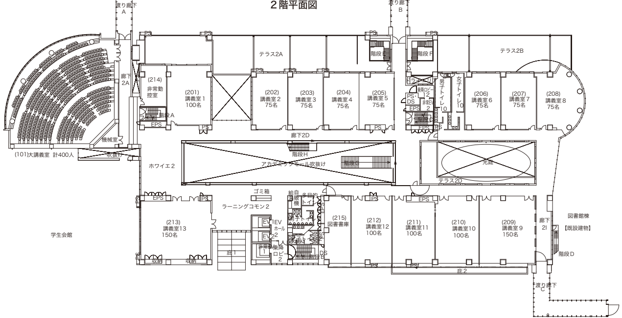
2階平面図
