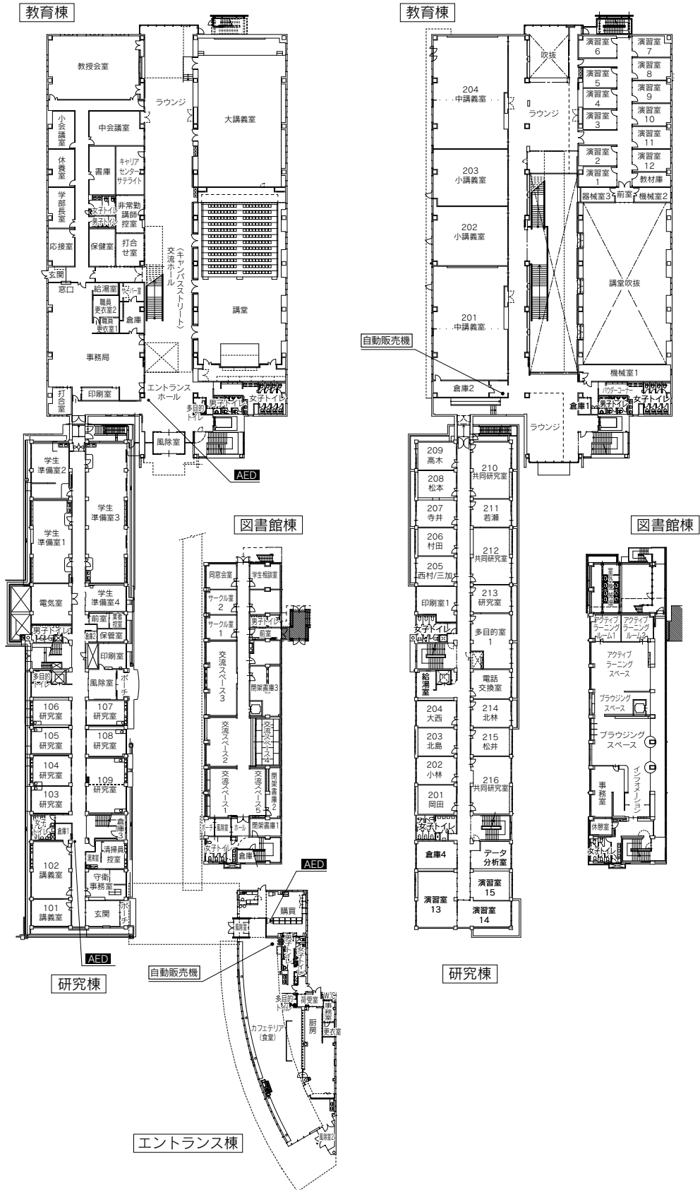
1階平面図
