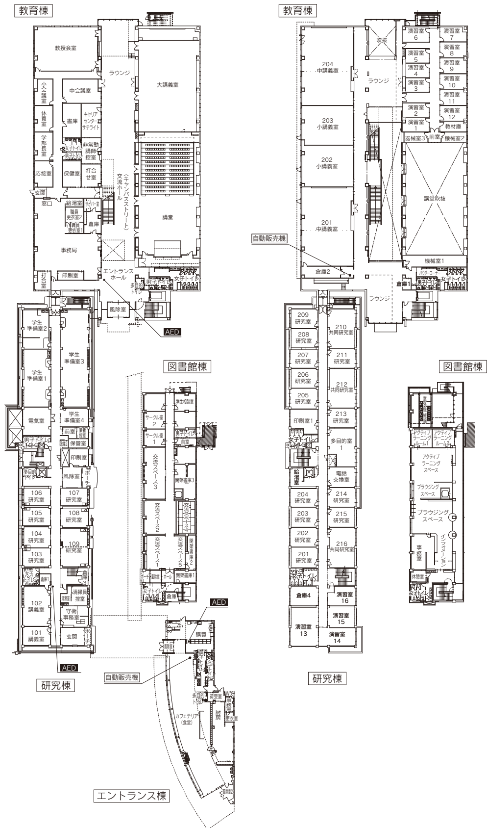
1階平面図
